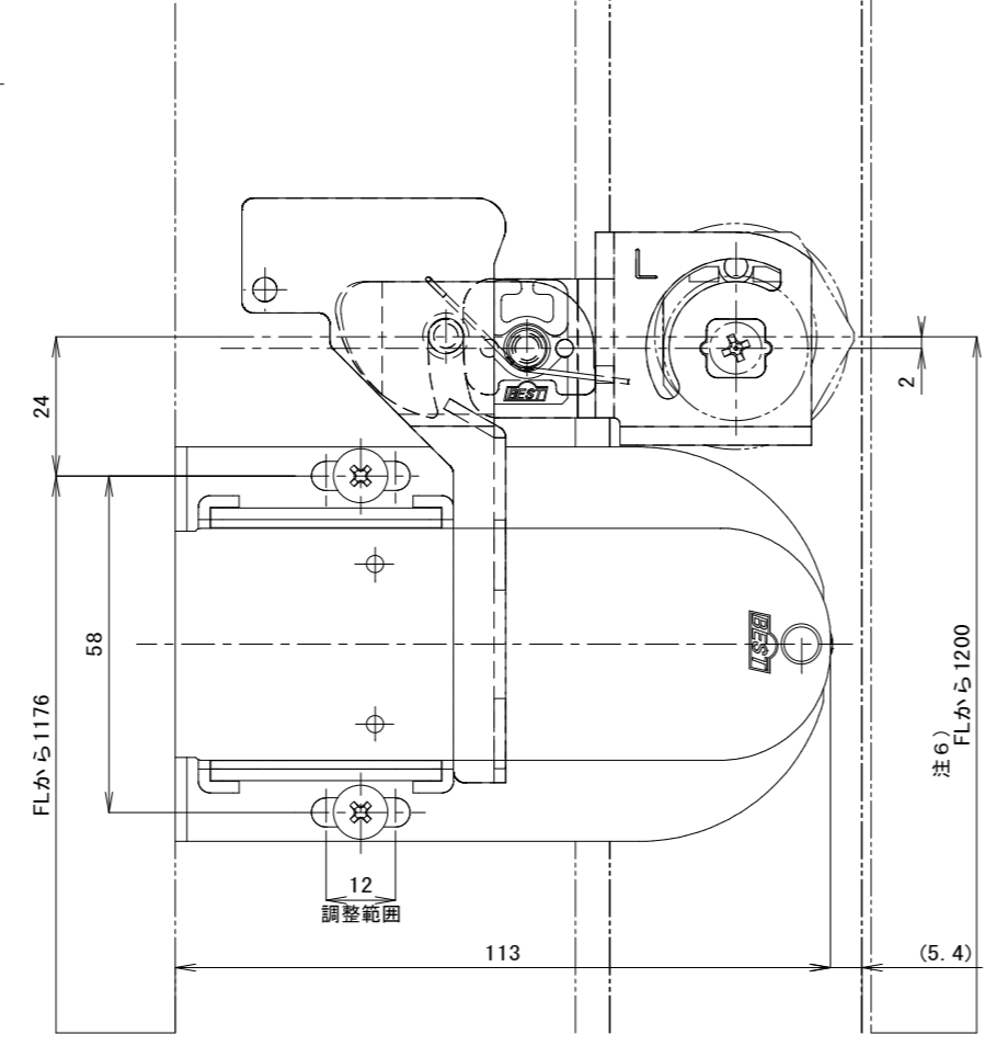
Dボード無し 納まり図
